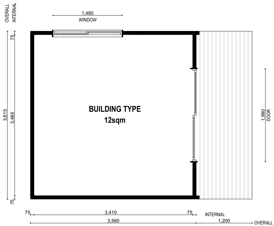
01 PLAN 1:50
