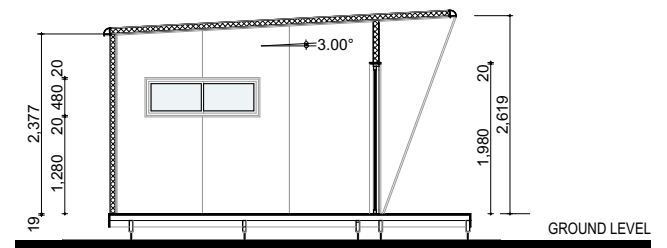
06 SECTION 1:100
