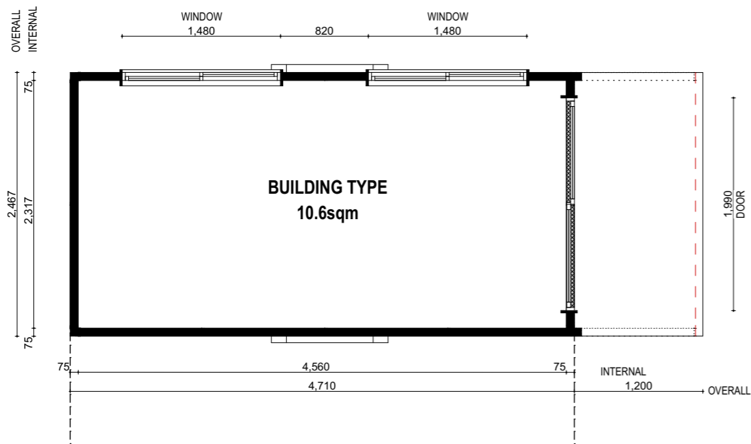
01 PLAN 1:50
