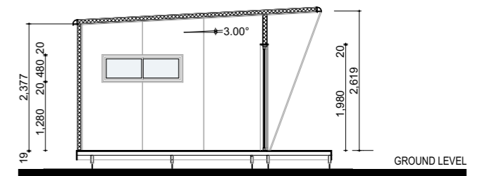
06 SECTION 1:100
