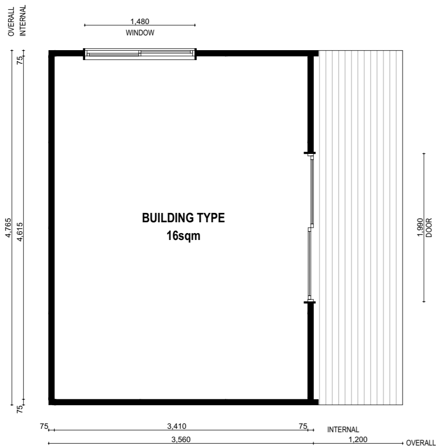
01 PLAN 1:50
